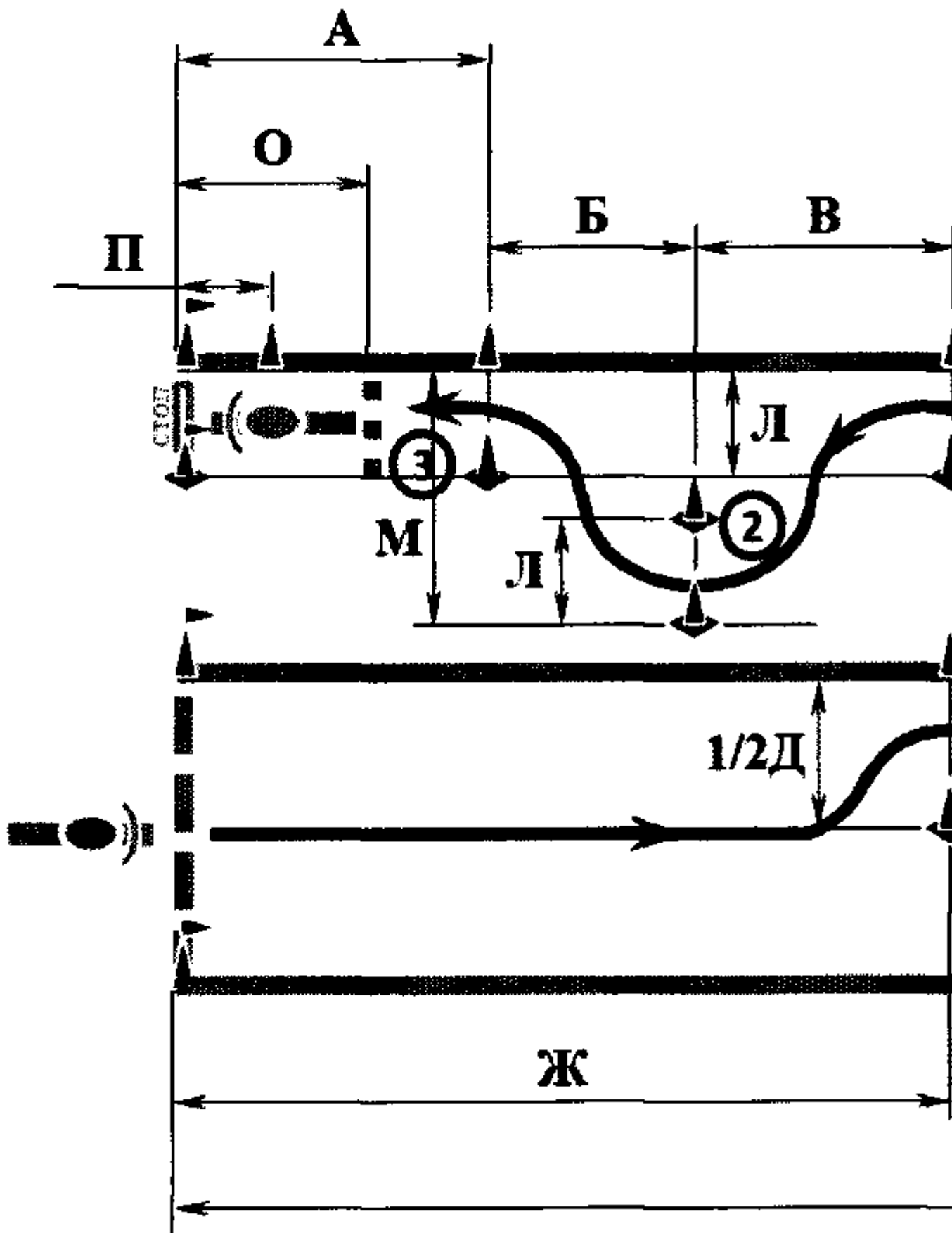
Рисунок 4. Схема "А" упражнения № 4
