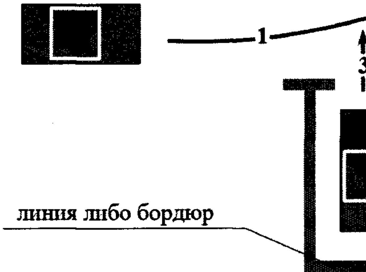
Рисунок 1. Схема маневра "Постановка транспортного средства на место стоянки при движении задним ходом с поворотом на 90 градусов"
